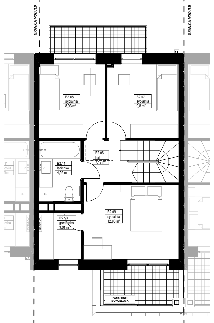
PIĘTRO
